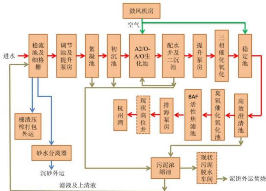
图 5.2-4 绍兴市上虞区水处理发展有限责任公司扩建项目污水处理工艺流程图
