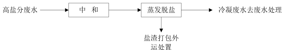
图 7.1-1 高盐分废水脱盐预处理工艺流程图
