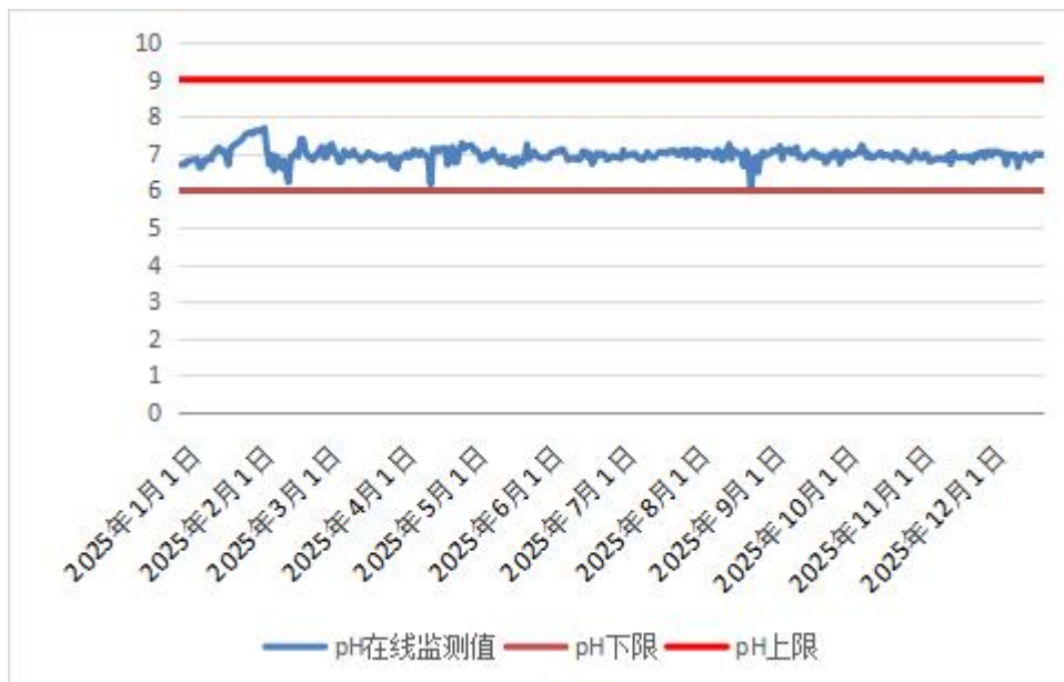
图 3.4.2-6 现有企业在线监测 pH 统计图
