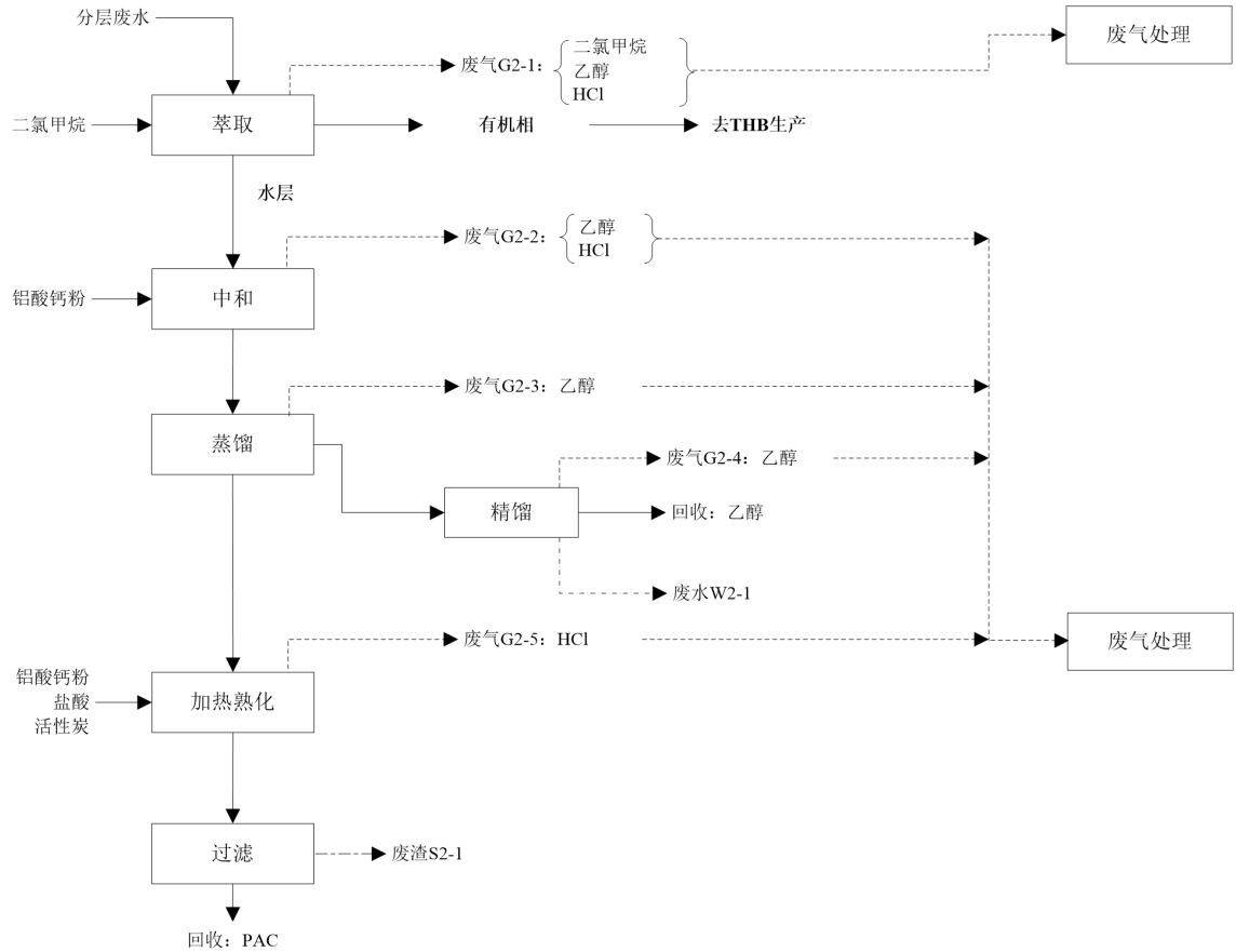
图 3.3.2.2-2 副产 PAC、乙醇回收工艺流程图
