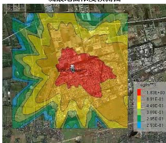
图 6.1.5-5 正常工况、全年逐日气象条件下硫酸地面浓度预测图
