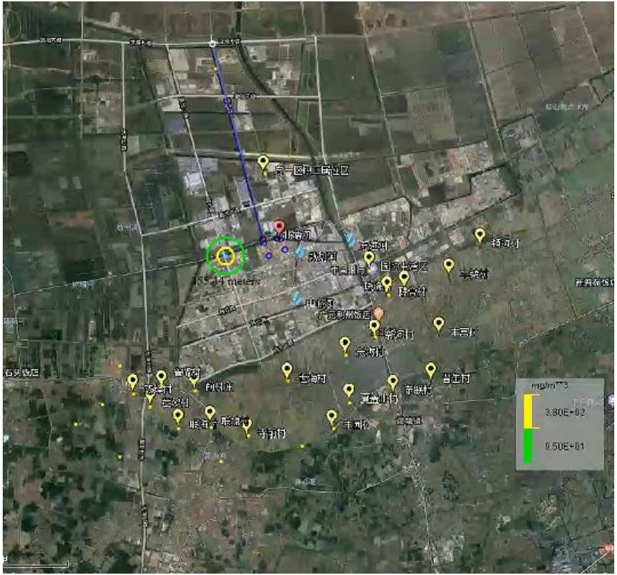
图 6.10.5-4 一氧化碳最常见气象条件下不同距离最大浓度
