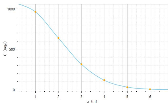
泄漏 30d 后 COD Mn 污染物运移范围图
