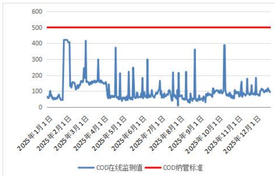
图 3.4.2-4 现有企业在线监测 CODcr 统计图（CODcr 单位：mg/L）
