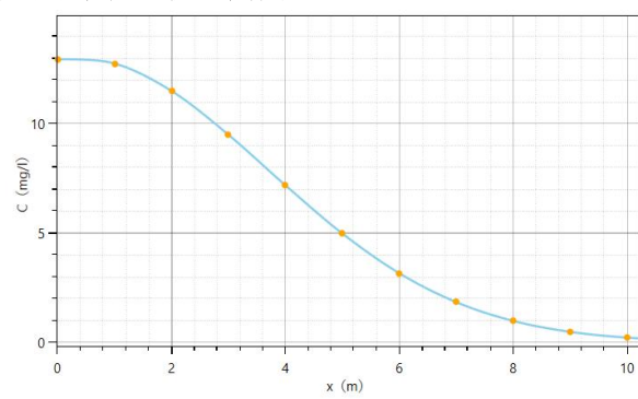
泄漏 100d 后氨氮污染物运移范围图
