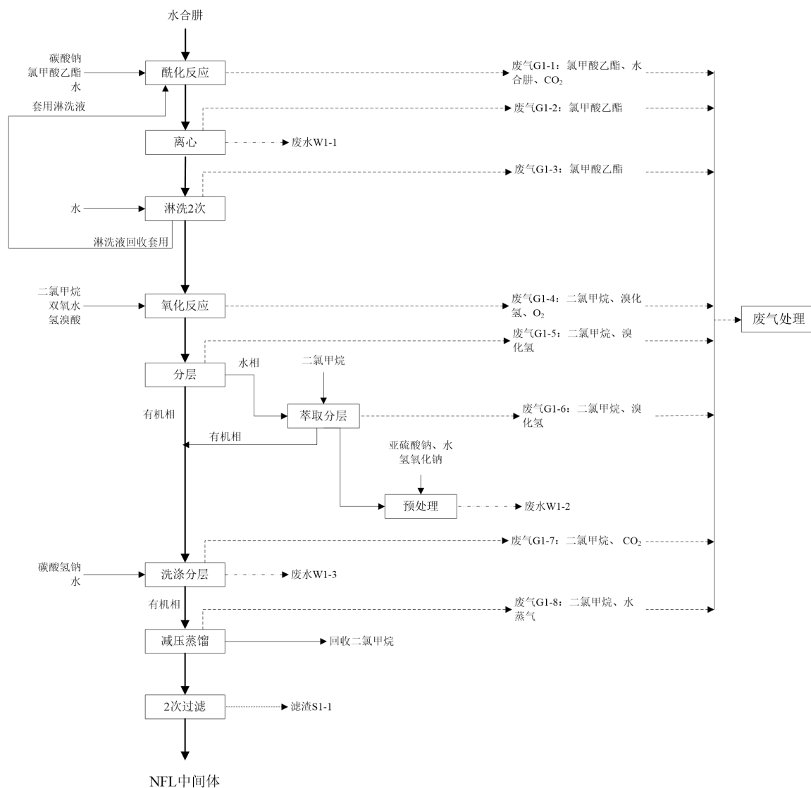
图3.3.2.3-1 NFL制备工段生产工艺流程图
