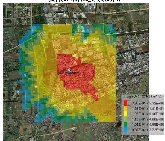
图 6.1.5-7 非正常工况、全年逐时气象条件下氨地面浓度预测图
