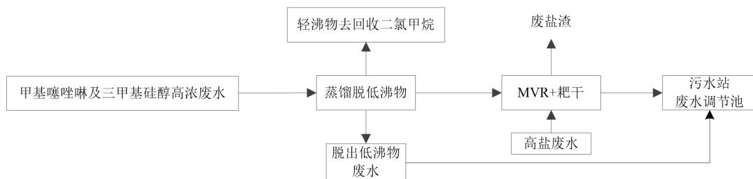
图 3.4.2-1 甲基噻唑啉生产线废水预处理工艺流程图
