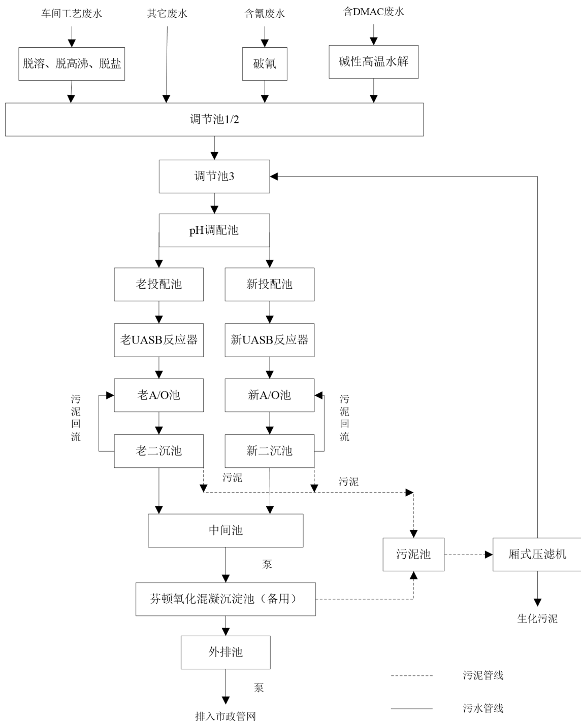
图 7.1-2 污水站处理工艺流程
