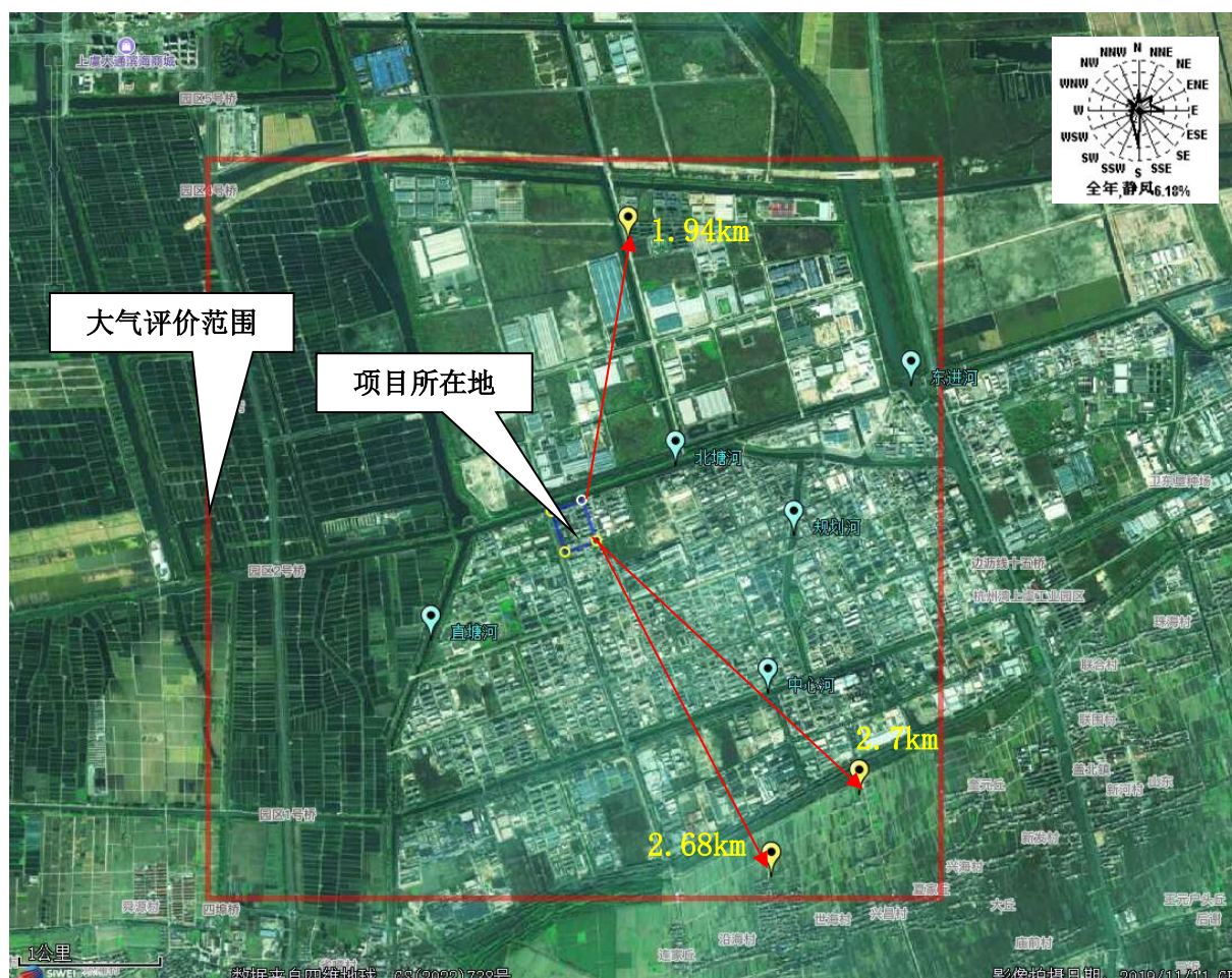
图 2.4-1 项目大气评价范围及主要保护目标分布图
