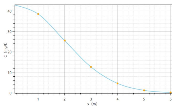
泄漏 30d 后氨氮污染物运移范围图
