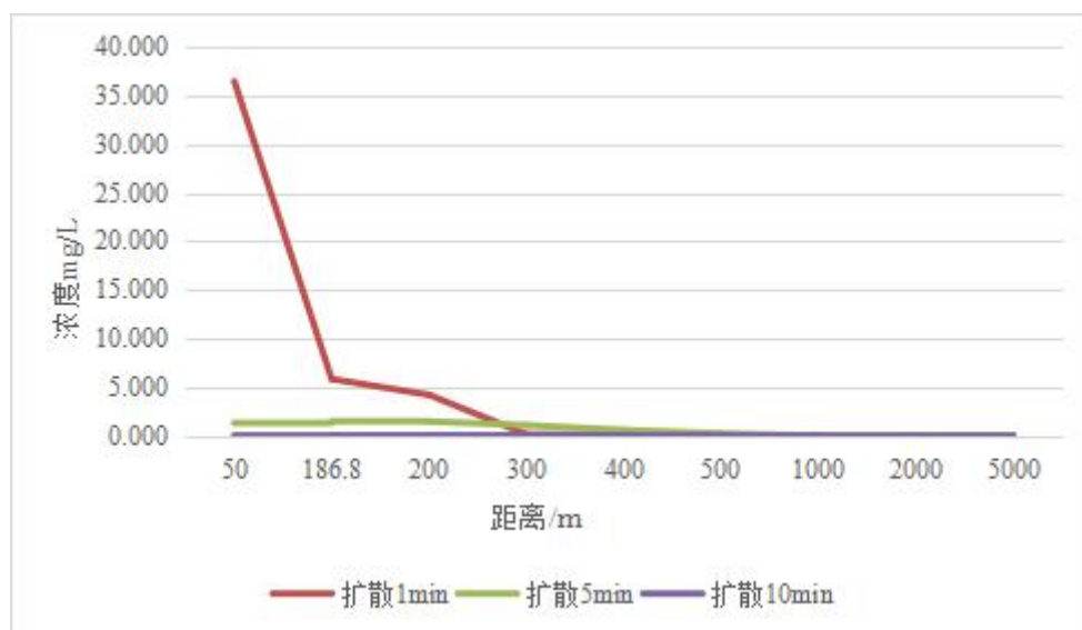
图 6.10.5-5 不同扩散时间下不同距离氨氮浓度变化图
