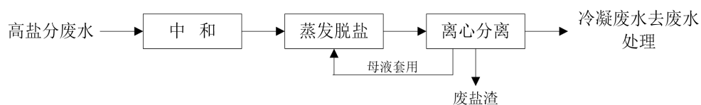
图 3.4.2-2 高盐分废水 MVR 脱盐预处理工艺流程图
