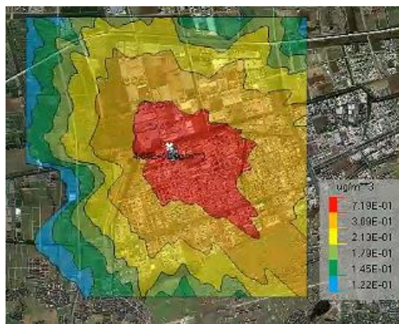
图 6.1.5-3 正常工况、全年逐时气象条件下硫酸地面浓度预测图
