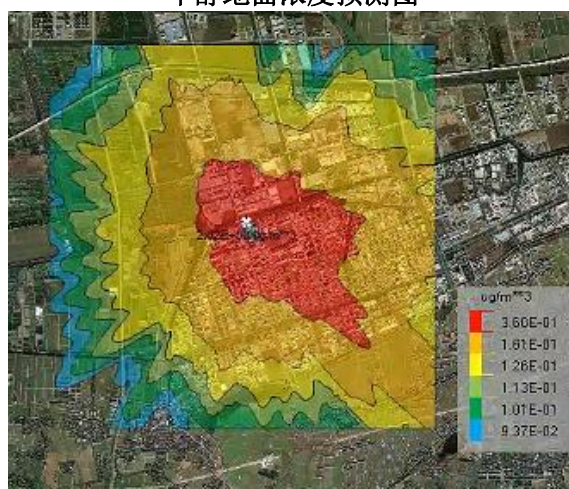
图 6.1.5-8 非正常工况、全年逐时气象条件下硫酸地面浓度预测图
