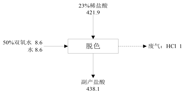
图 3.3.2.3-4 副产盐酸回收工艺流程图
