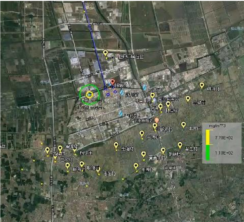
图6.10.5-1 氨最不利气象条件下不同距离最大浓度
