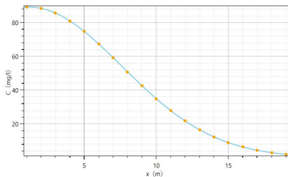
泄漏 365d 后 COD Mn 污染物运移范围图
