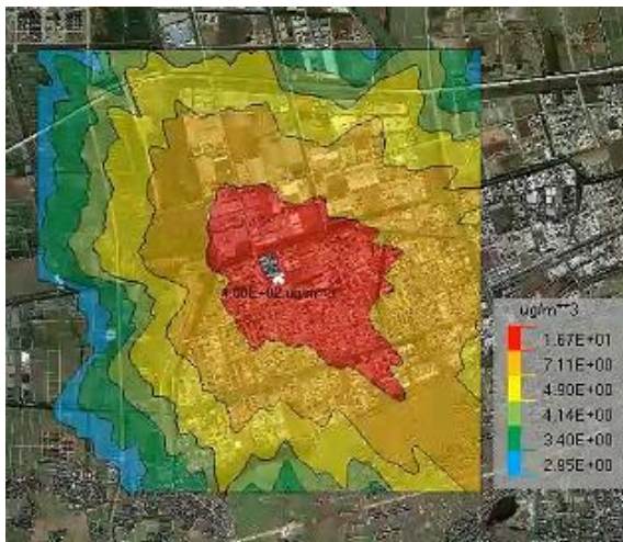
图 6.1.5-1 正常工况、全年逐时气象条件下 甲醇地面浓度预测图
