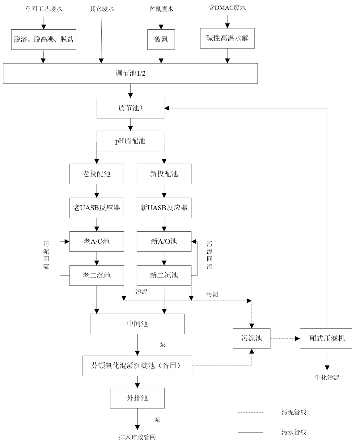
图 3.4.2-3 现有污水站处理工艺流程
