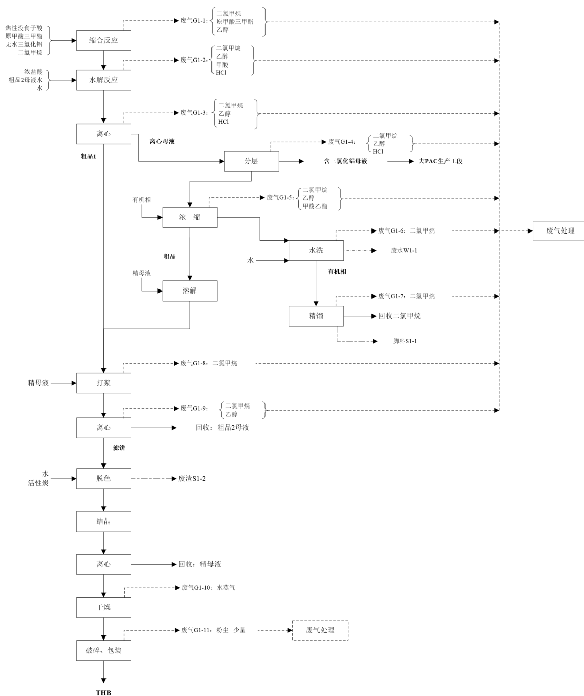
图 3.3.2.2-1 THB 生产工艺流程图
