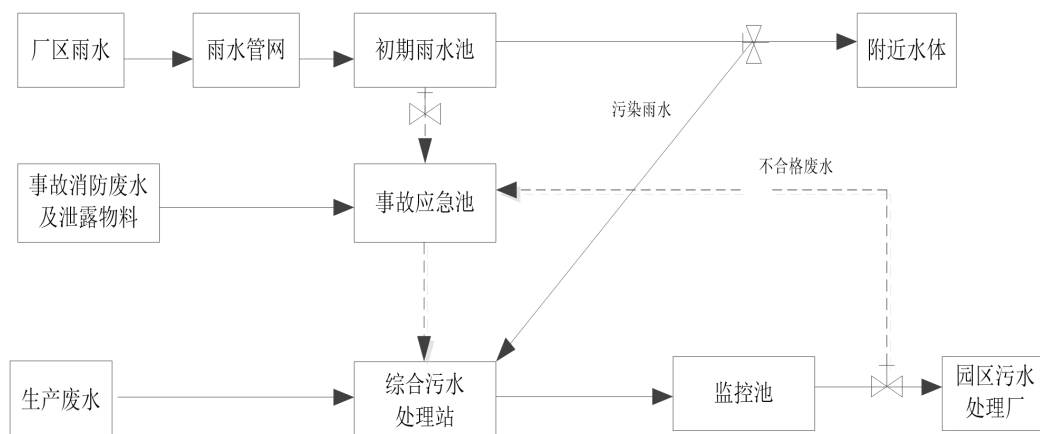
图 6.10.6-4 本项目事故水收集系统流程示意图
