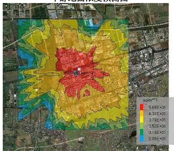
图 6.1.5-6 非正常工况、全年逐时气象条件下甲醇地面浓度预测图
