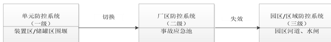
图 6.10.6-3 事故水三级防控系统流程示意图
