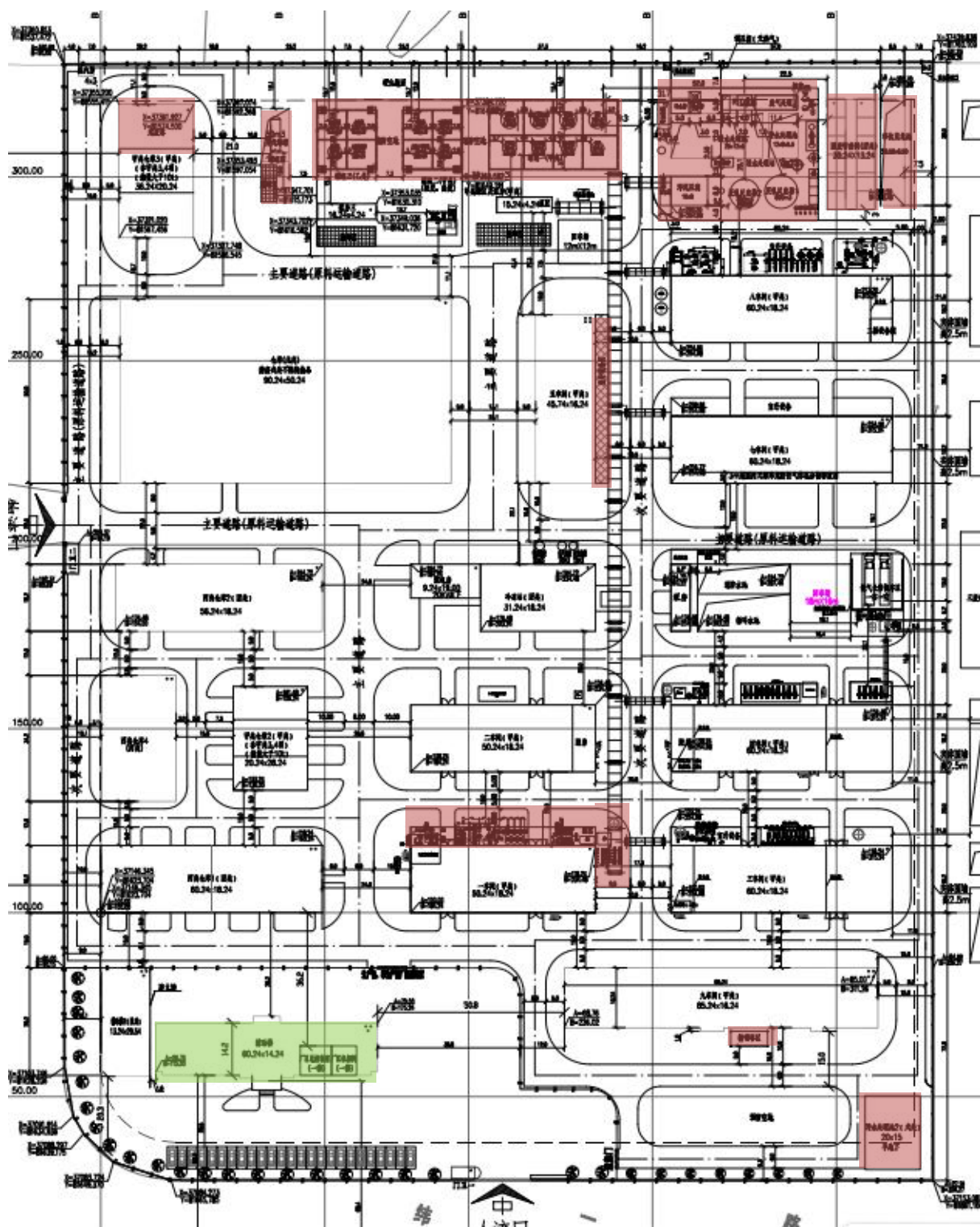
注：红色区域属重点防渗区、绿色区域属简单防渗区、未标注部分属一般防渗区。 图 7.3-1 分区防渗图
