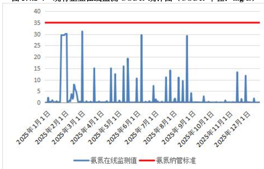
图 3.4.2-5 现有企业在线监测氨氮统计图
