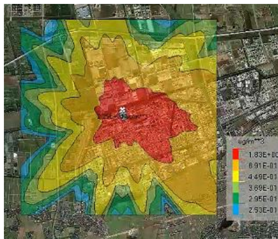
图 6.1.5-4 正常工况、全年逐日气象条件下甲醇地面浓度预测图
