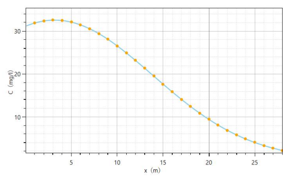
泄漏 1000d 后 COD Mn 污染物运移范围图
