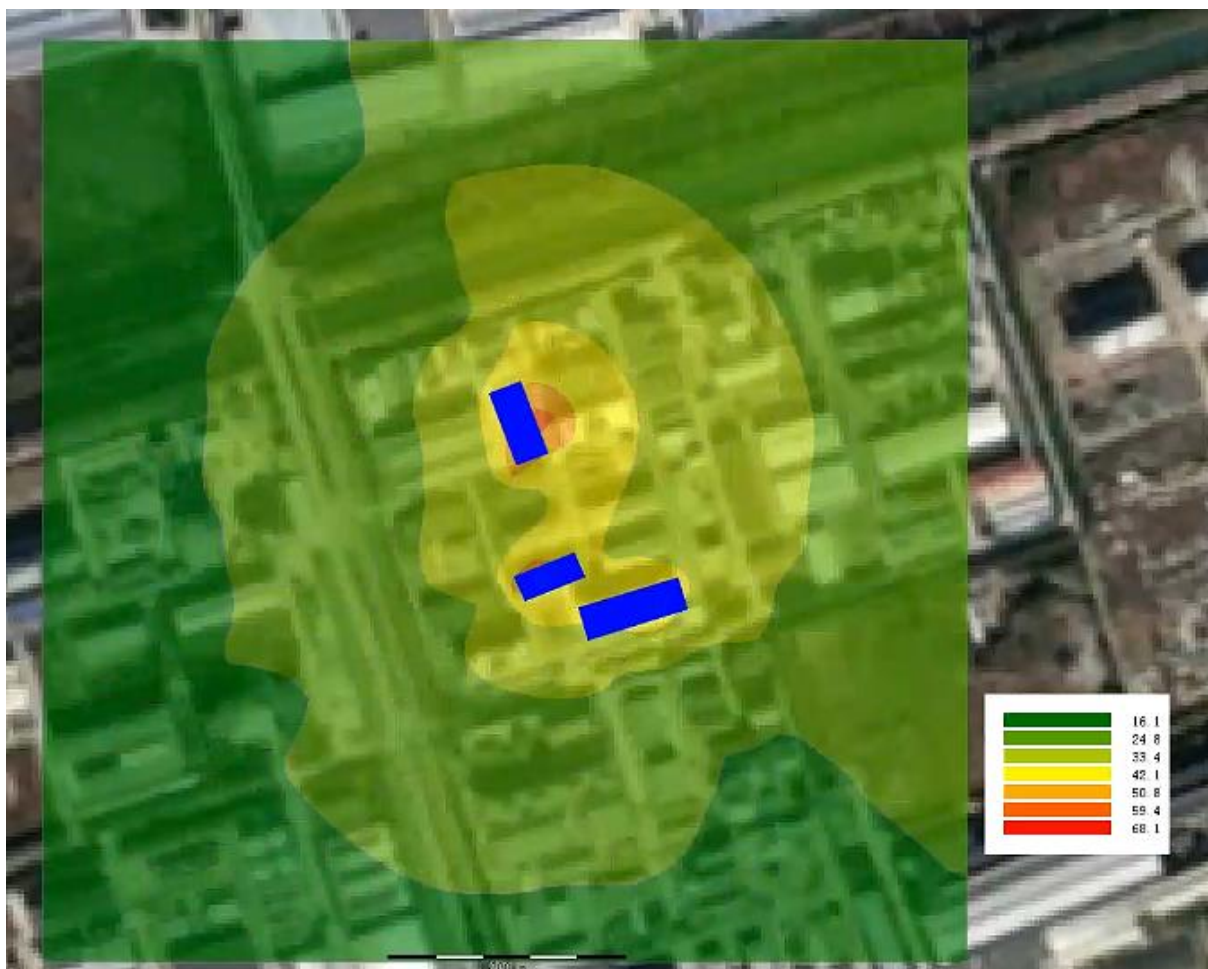
图 6.5-1 声环境影响预测结果图-贡献值
