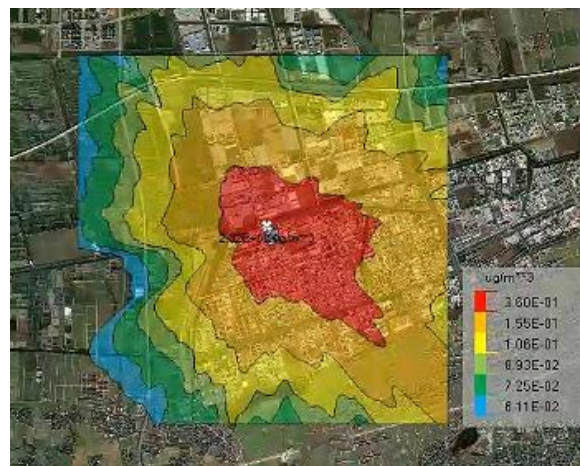
图 6.1.5-2 正常工况、全年逐时气象条件下 氨地面浓度预测图
